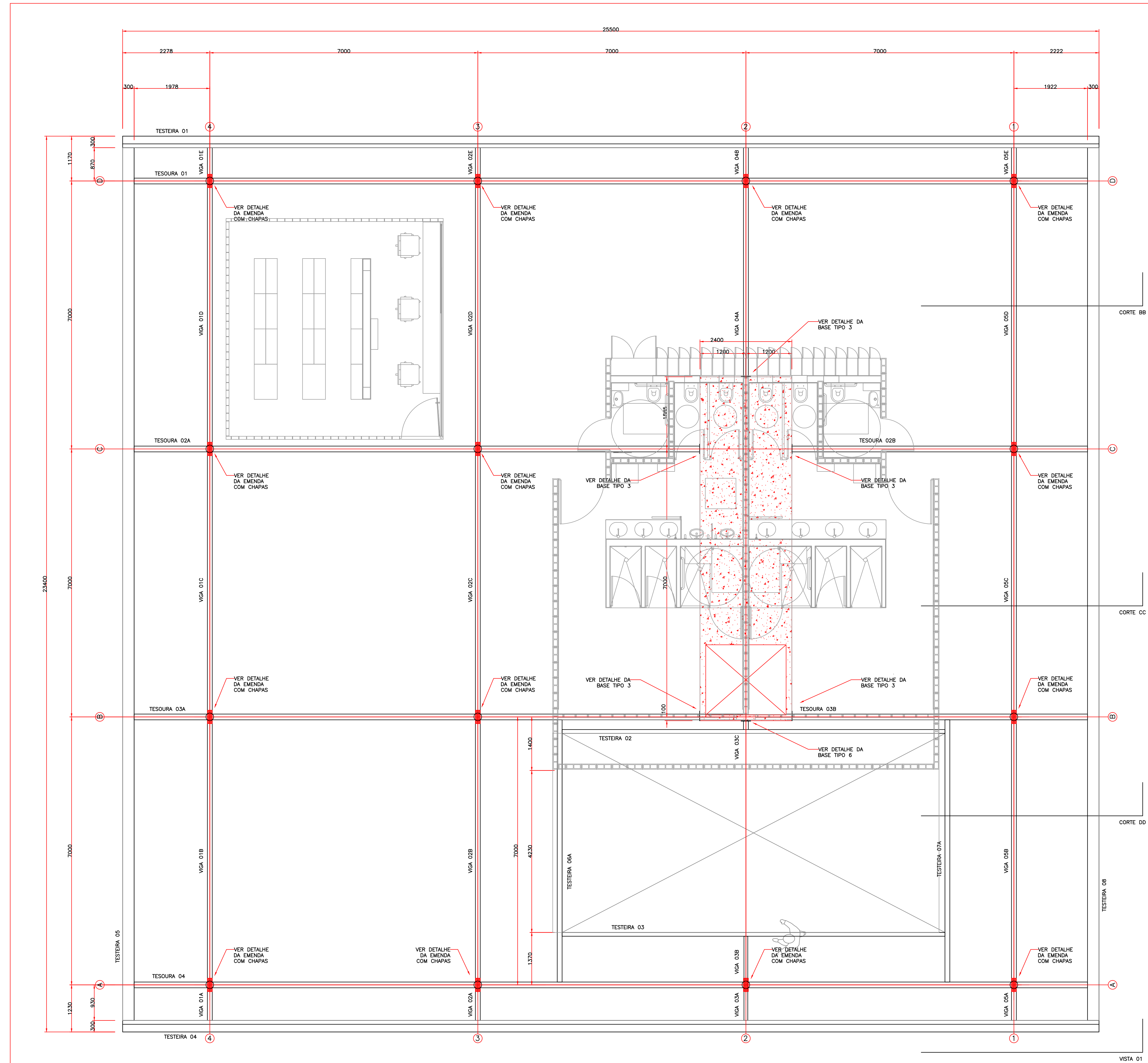
MONTAGEM DAS TESOURAS, VIGAS E TESTEIRAS DA COBERTURA ESC 1:50
