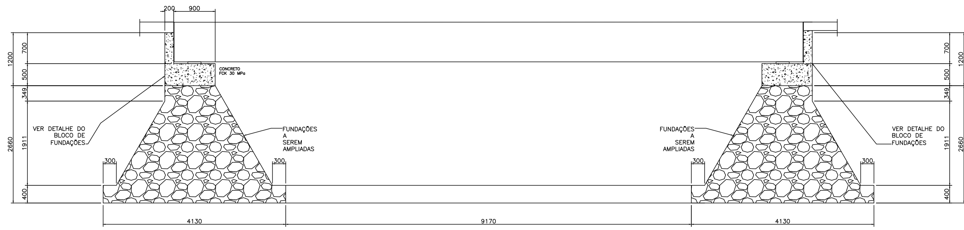
2 CORTE - FUNDAÇÕES ESCALA 1:500
