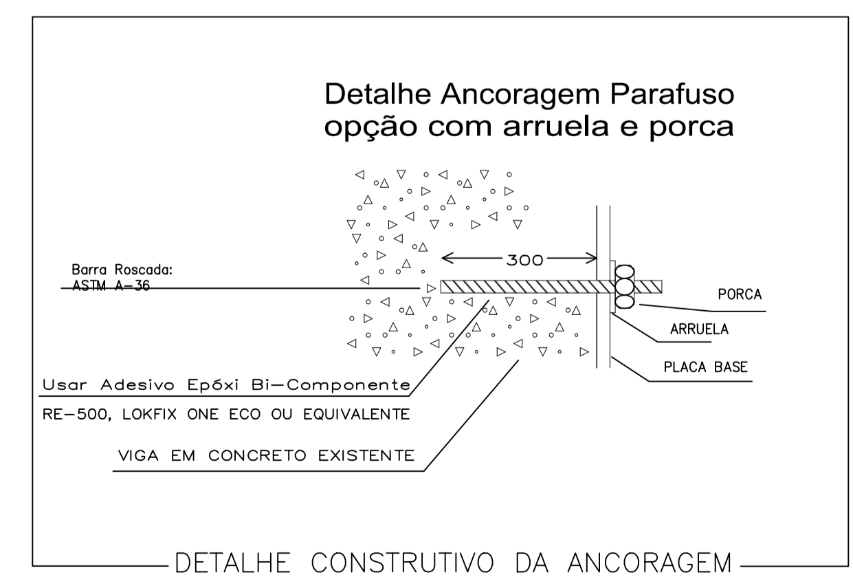
DET. TÍPICO EXECUÇÃO FIX. ADESIVO EPOXI s/ esc.
