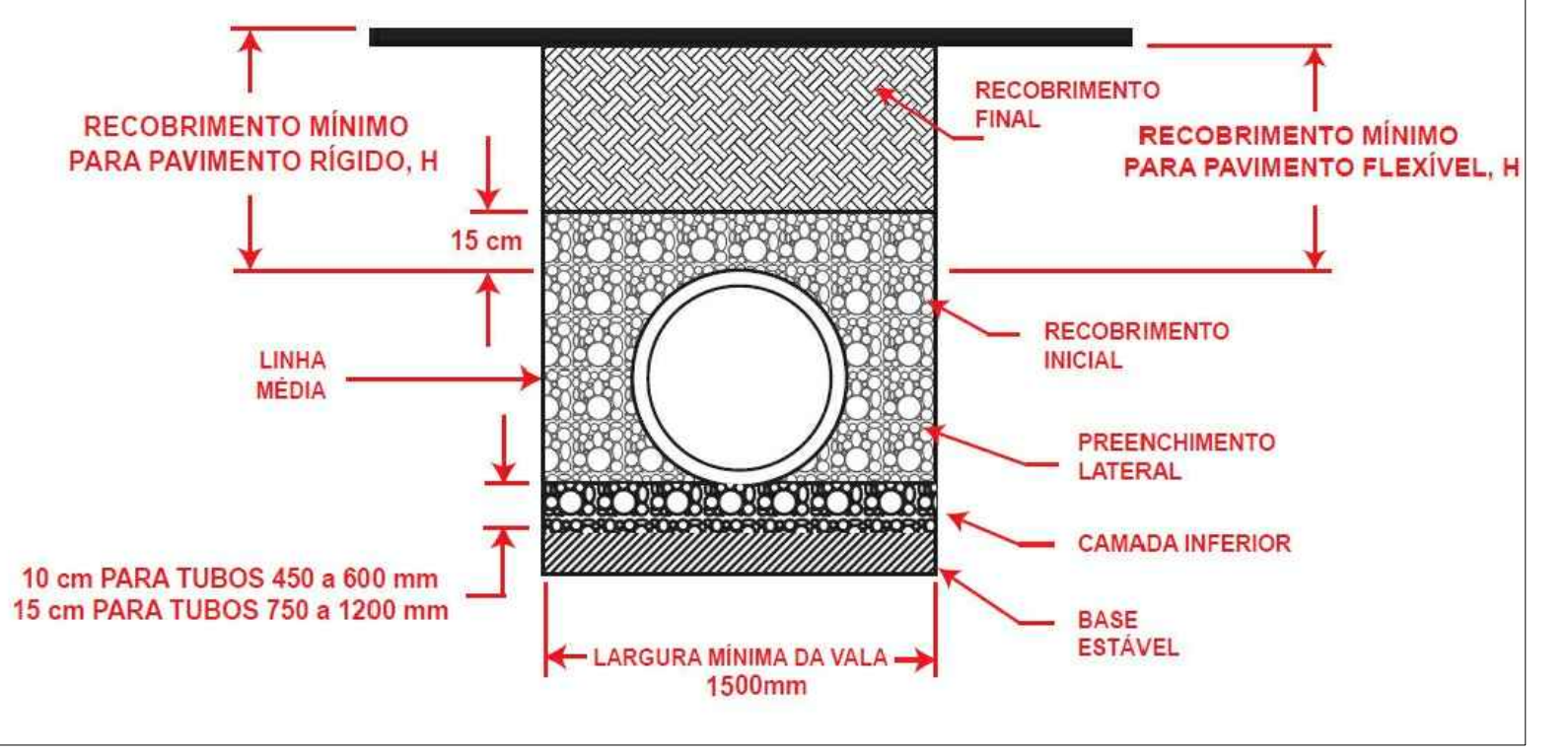
2 DETALHE DA VALA DE ASSENTAMENTO TUBO PEAD S/ESCALA
