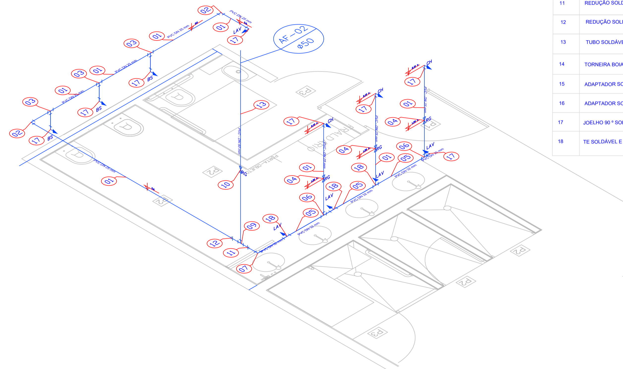
3 ESQUEMA DE ISOMETRICO ÁGUA FRIA - BWC FEM ESCALA 1:25
