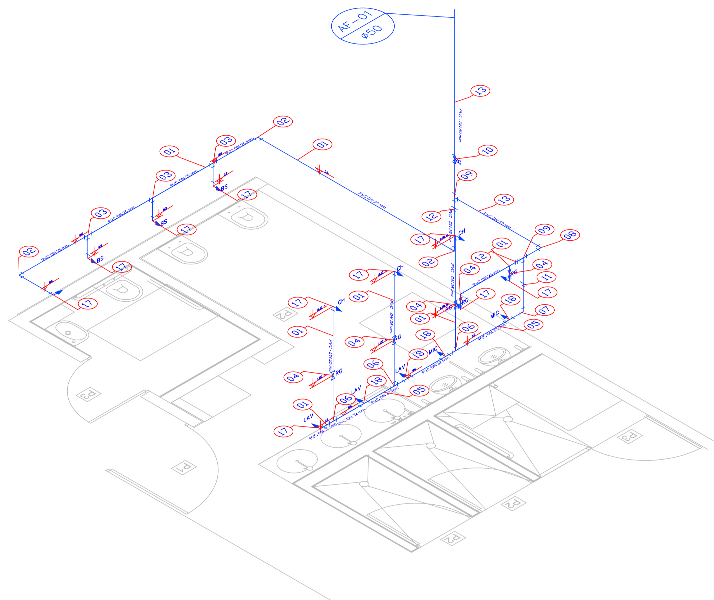
2 ESQUEMA DE ISOMETRICO ÁGUA FRIA - BWC MASC ESCALA 1:25
