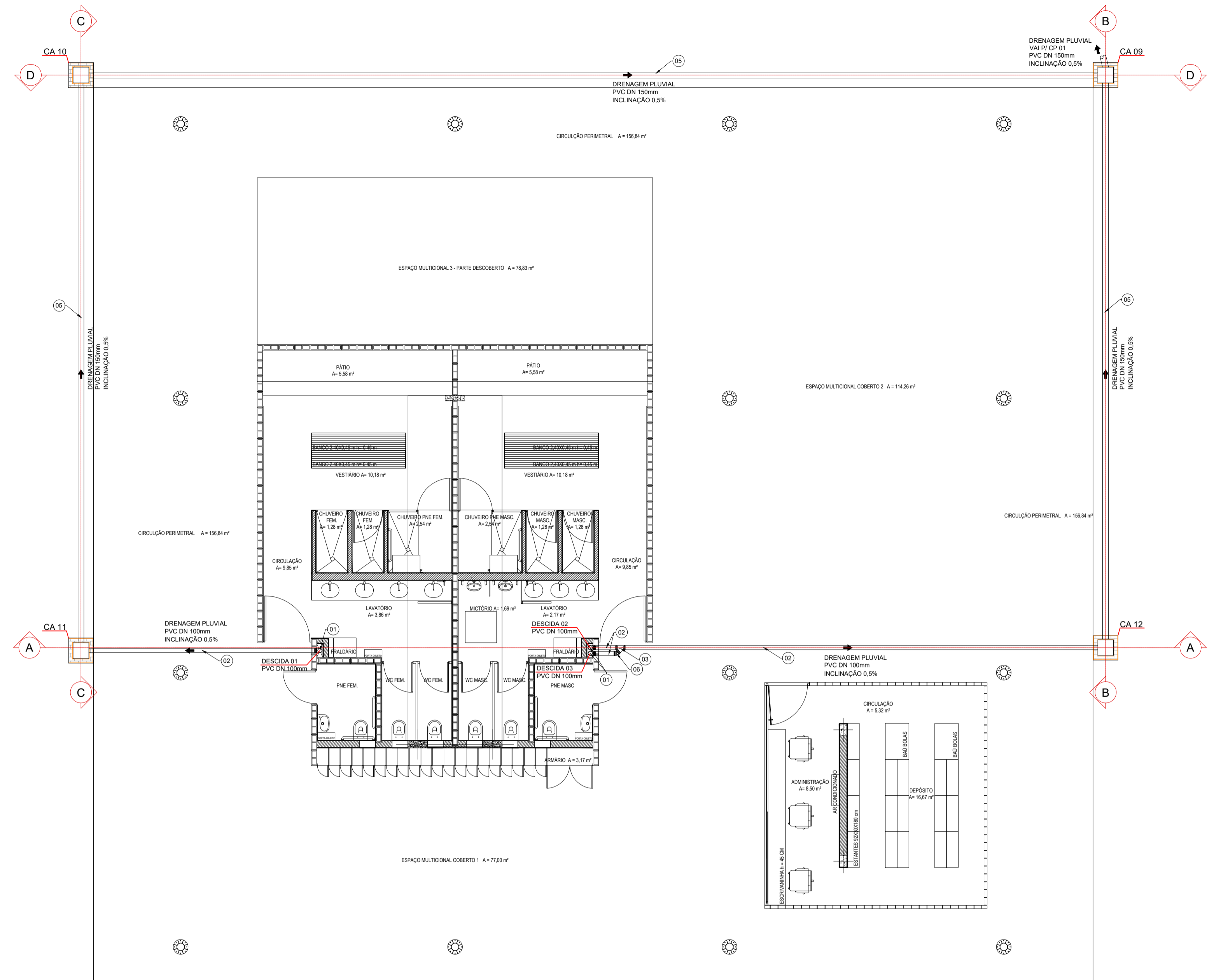
2 PLANTA BAIXA ESCALA 1:75
