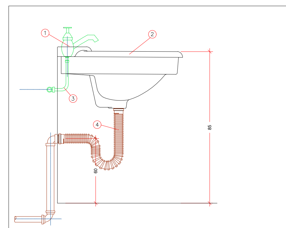
5 DETALHE LAVATÓRIO SEM ESCALA
