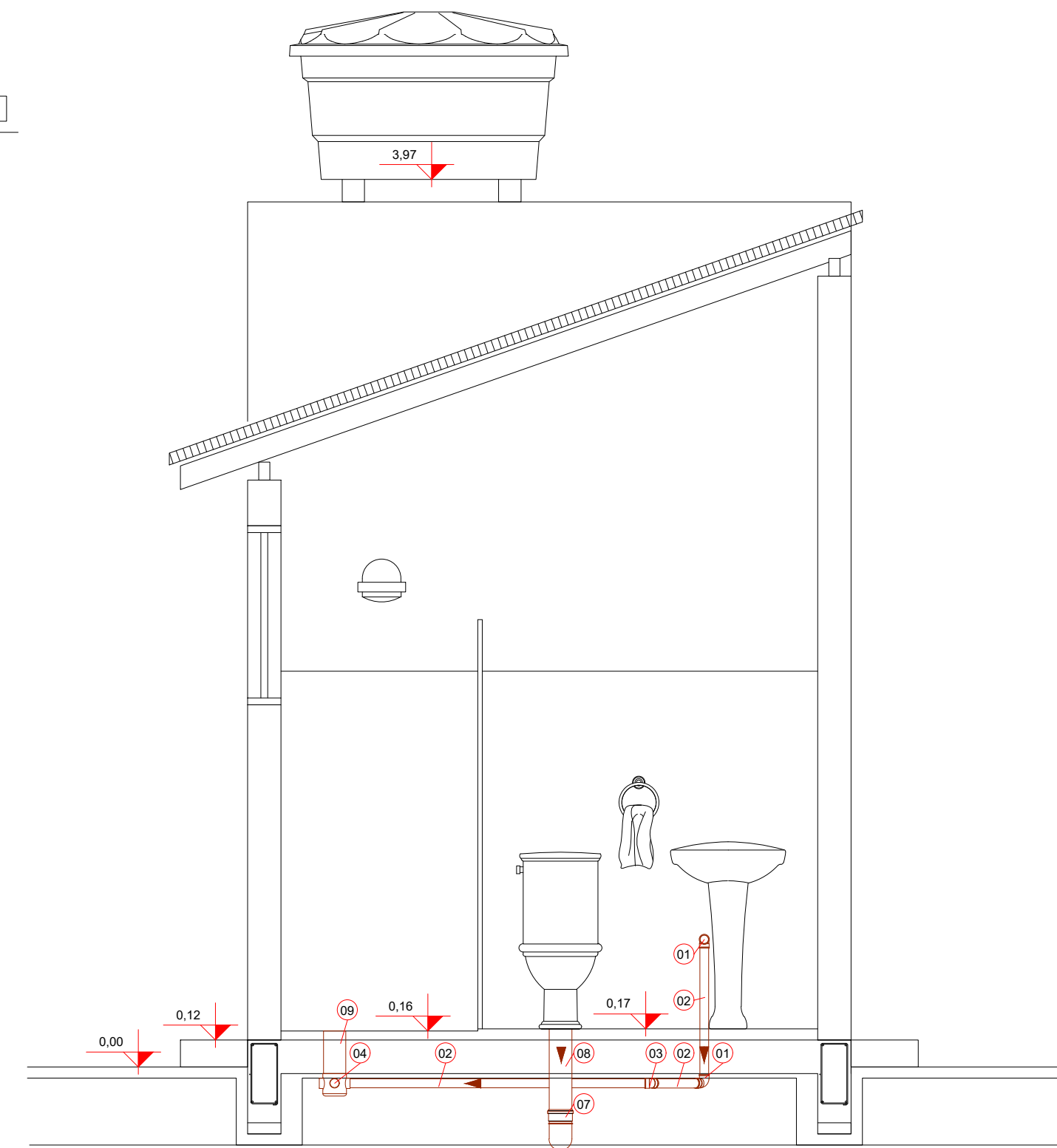
2 CORTE AA ESCALA 1:25
