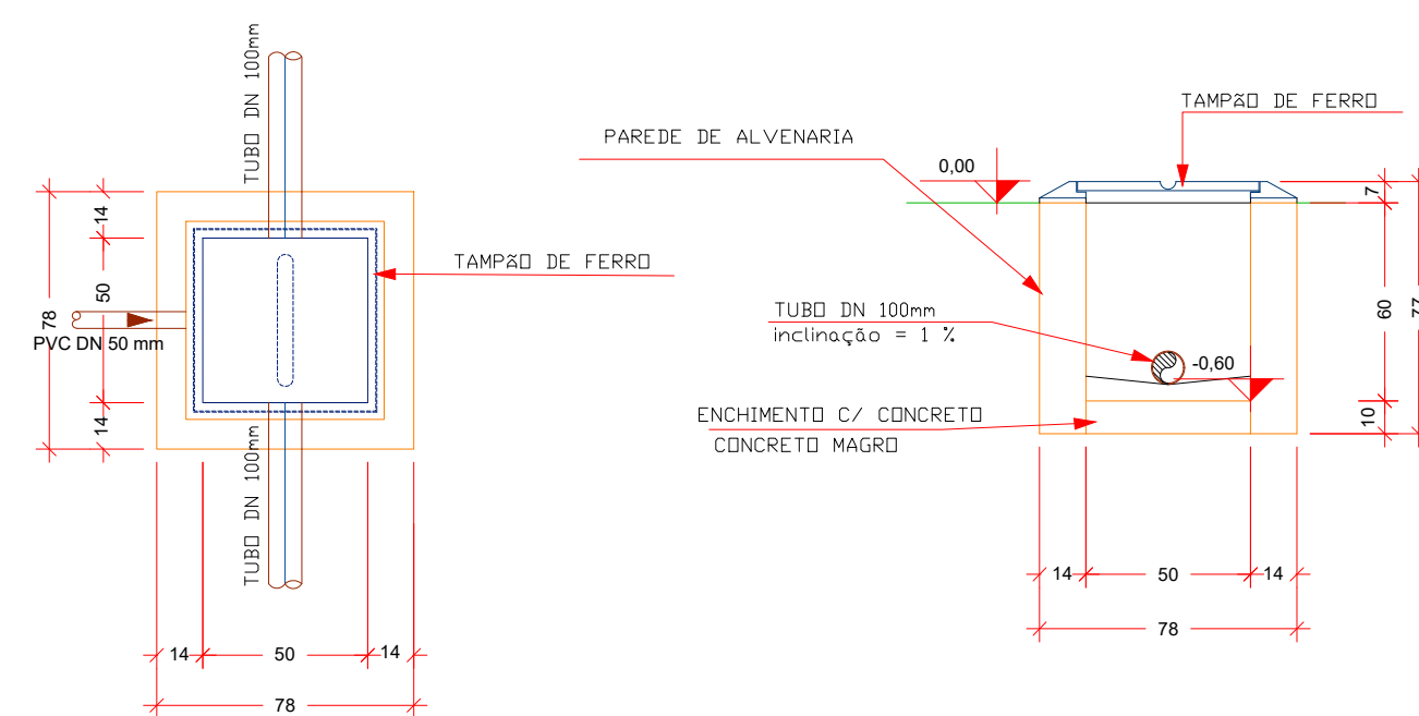
4 DETALHES DA CAIXA DE INSPEÇÃO ESCALA 1:20
