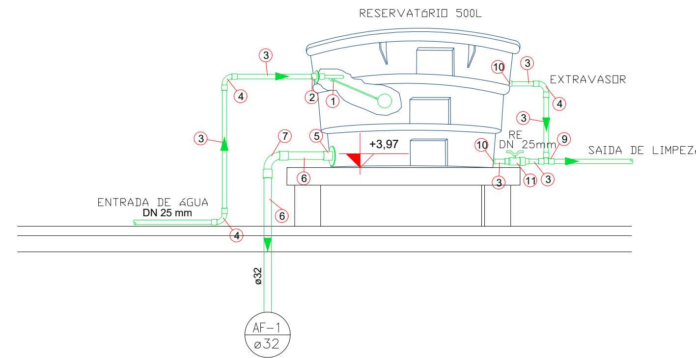
2 DETALHES CAIXA D'ÁGUA ESCALA 1:20
