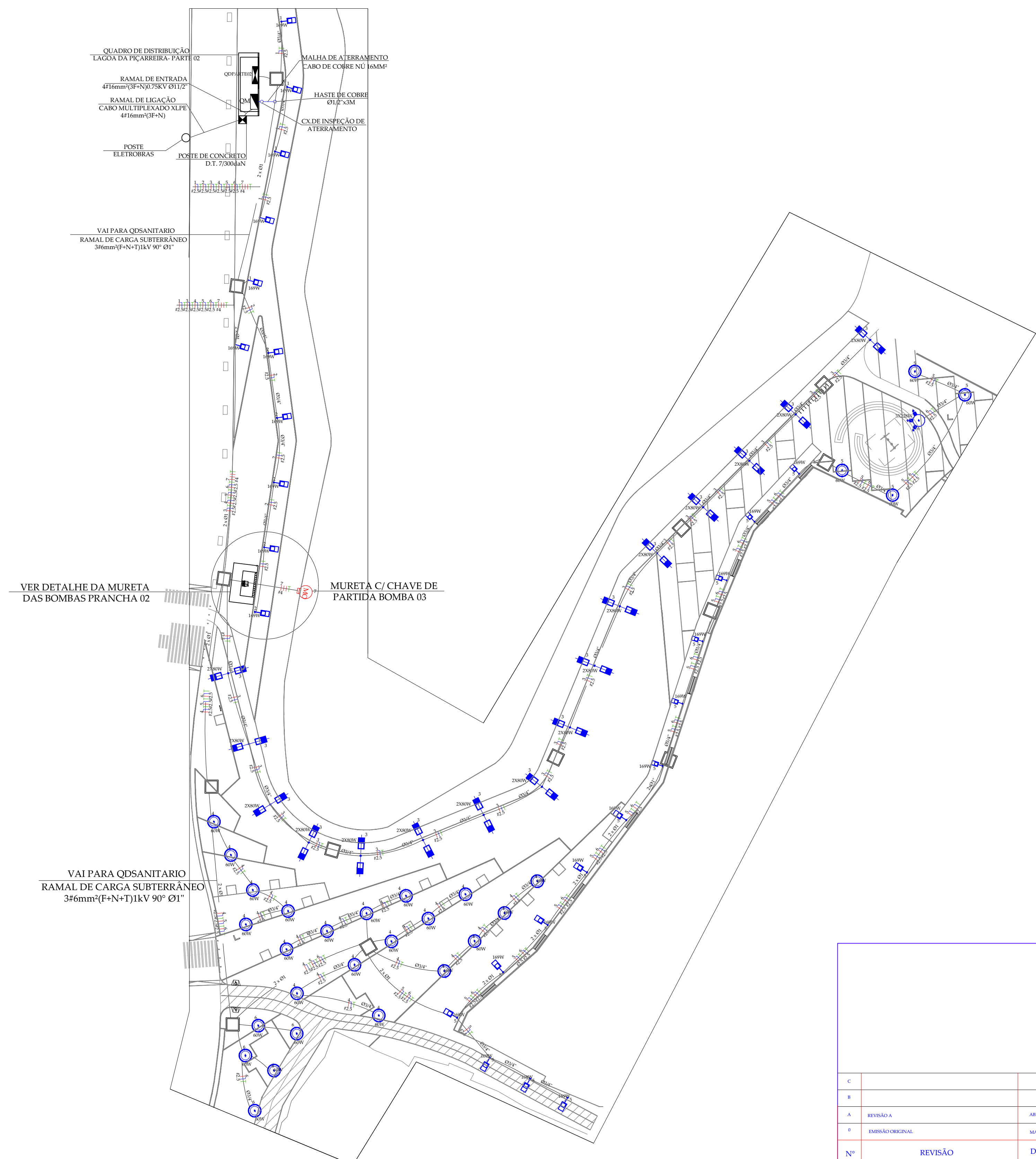
DIST. ELÉTRICA - PIÇARREIRA - PARTE 02 ESC.: 1/600
