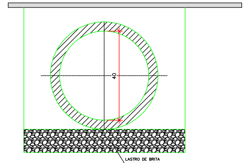
GALERIA - BSTC Ø 40 - CORTE TRANSVERSAL
