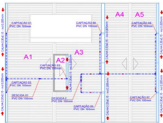
Figura 01 - Distribuição de áreas de contribuição, posicionamento de calhas coletoras e dutos verticais
