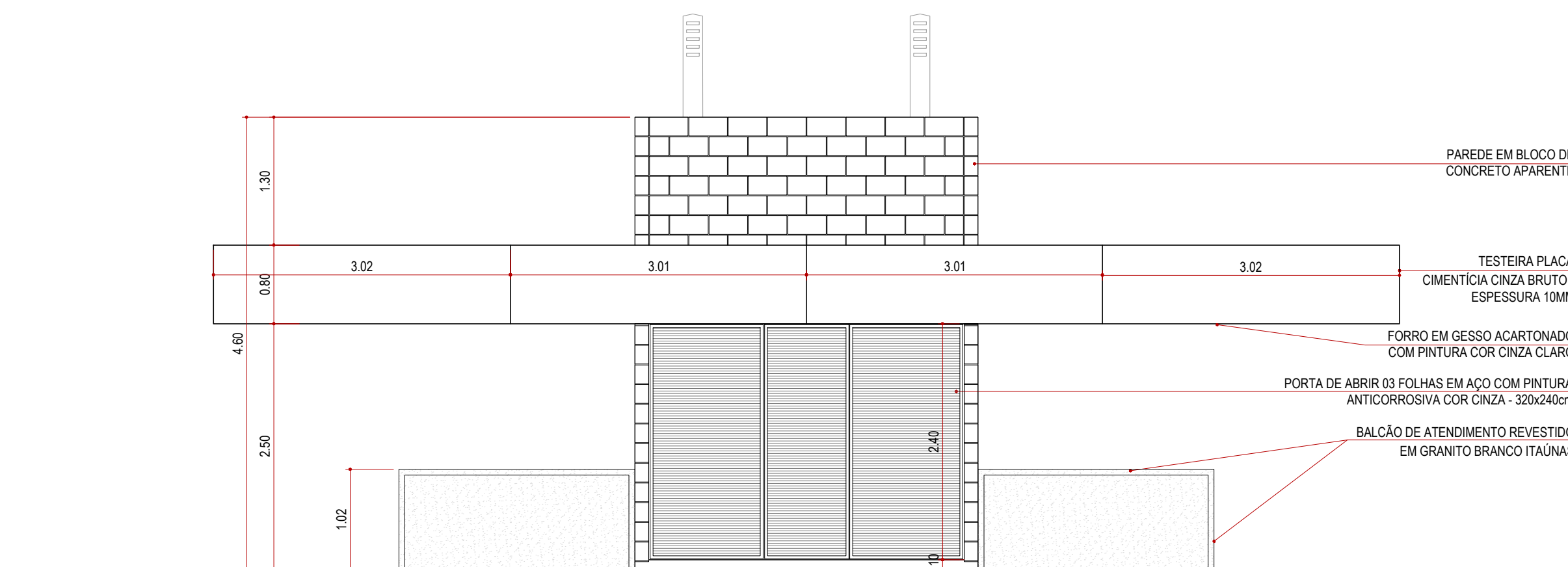
ELEVAÇÃO 2 - QUIOSQUE ABERTO ESCALA 1:50
