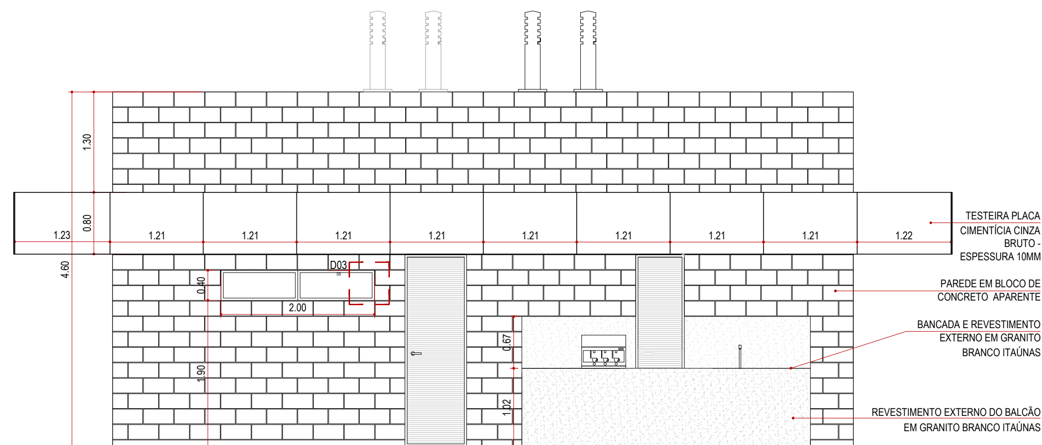
ELEVAÇÃO 1 - QUIOSQUE ABERTO ESCALA 1:50
