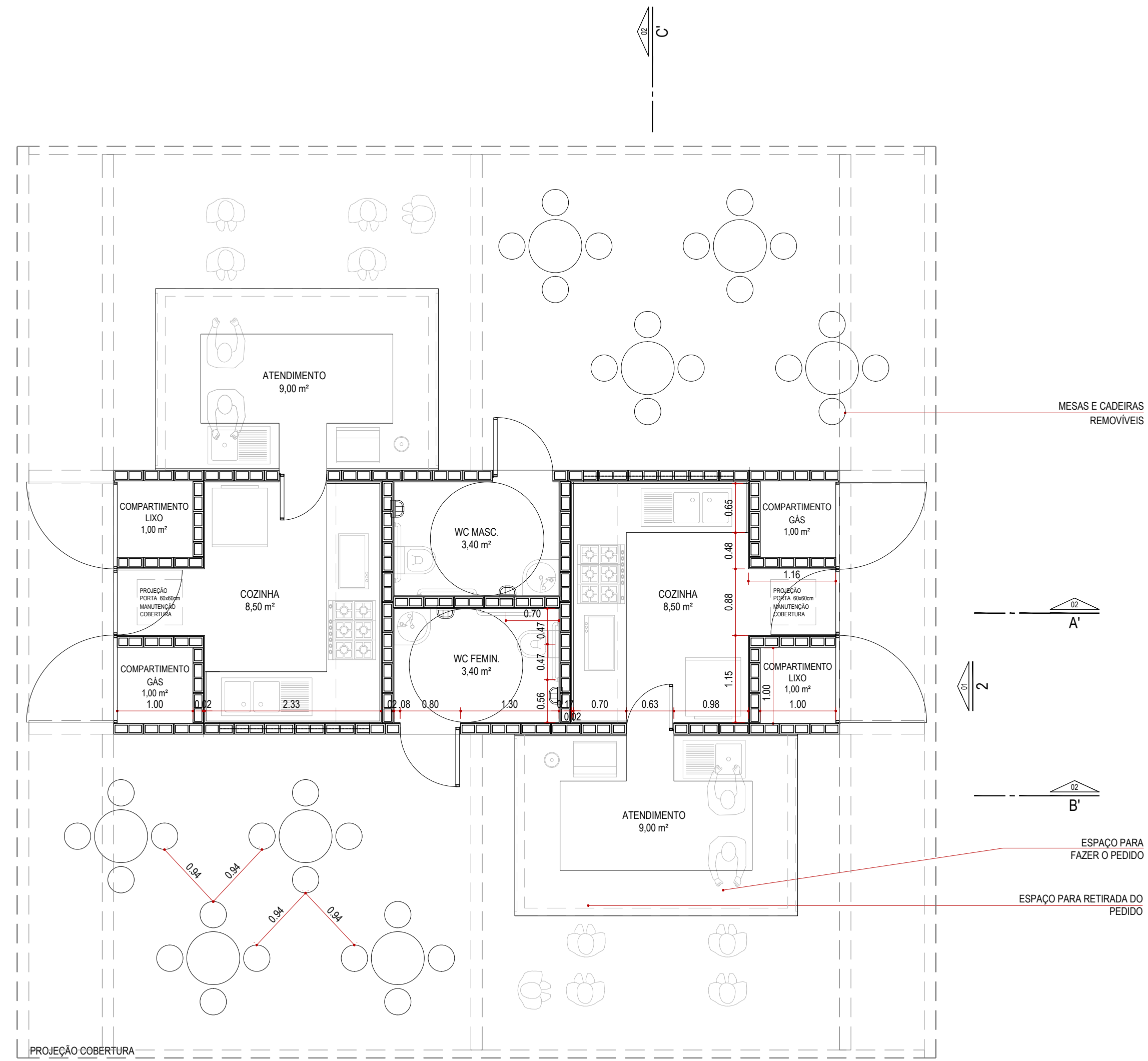
PLANTA LAYOUT MESAS E ATENDIMENTO - MODELO 2 ESCALA 1:50
