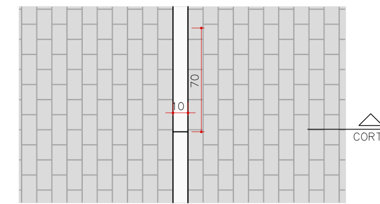
ENCONTRO DE PISOS - ENCONTRO DE RIOS - E9 PLANTA ESCALA 1:25
