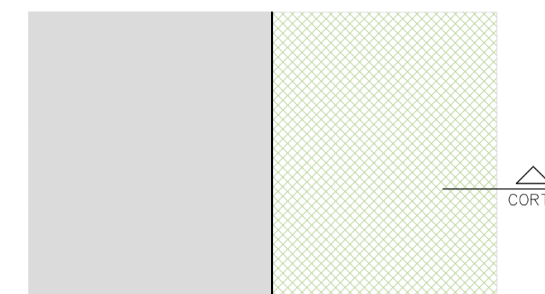
ENCONTRO DE PISOS - CONCRETO X GRAMA - E13 PLANTA ESCALA 1:25
