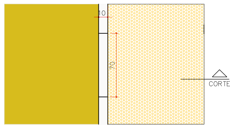
ENCONTRO DE PISOS - SOLO CIMENTO X GUIA X PEDRISCO - E7 PLANTA ESCALA 1:25
