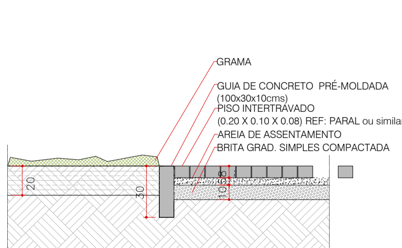
ENCONTRO DE PISOS - GRAMA X INTERTRAVADO - E15 CORTE ESCALA 1:25
