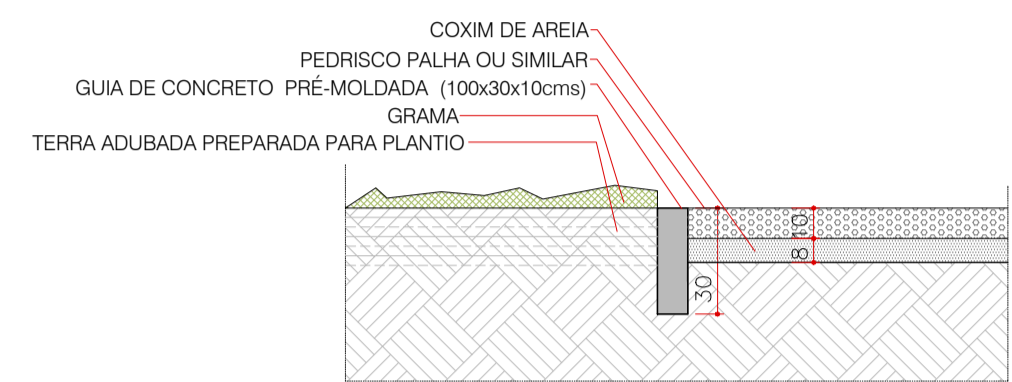
ENCONTRO DE PISOS - GRAMA X GUIA X PEDRISCO - E8 CORTE ESCALA 1:25
