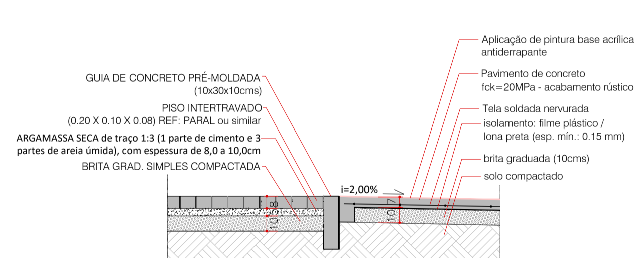
ENCONTRO DE PISOS - SOLO CIMENTO X CICLOVIA - E14 CORTE ESCALA 1:25
