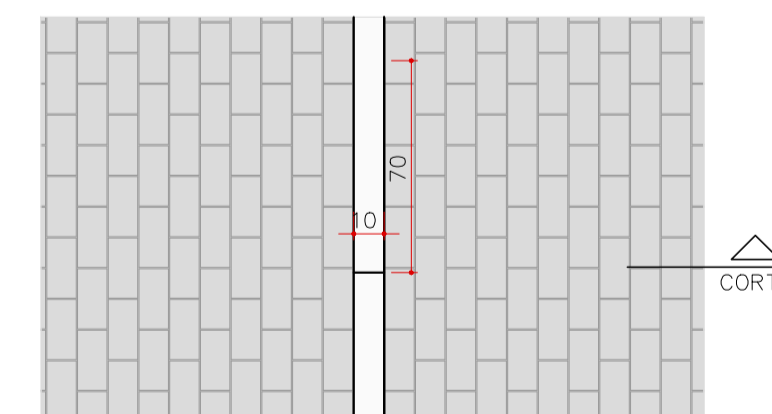
ENCONTRO DE PISOS - VIA DE INTERTRAVADO - E17 PLANTA ESCALA 1:25
