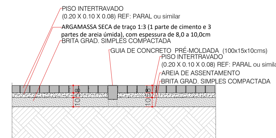
ENCONTRO DE PISOS - ENCONTRO DE RIOS - E9 CORTE ESCALA 1:25
