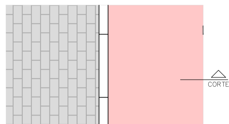
ENCONTRO DE PISOS - INTERTRAVADO X CICLOVIA - E14 PLANTA ESCALA 1:25
