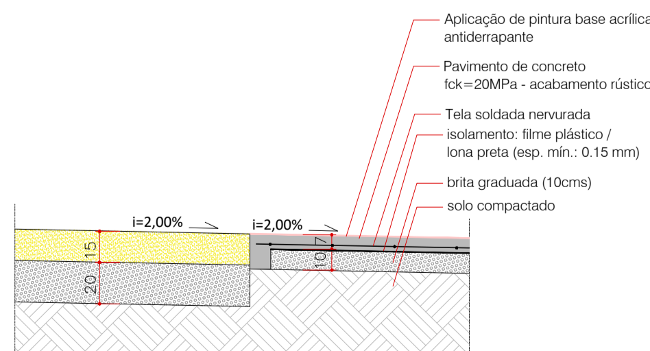
ENCONTRO DE PISOS - SOLO CIMENTO X CICLOVIA - E16 CORTE ESCALA 1:25
