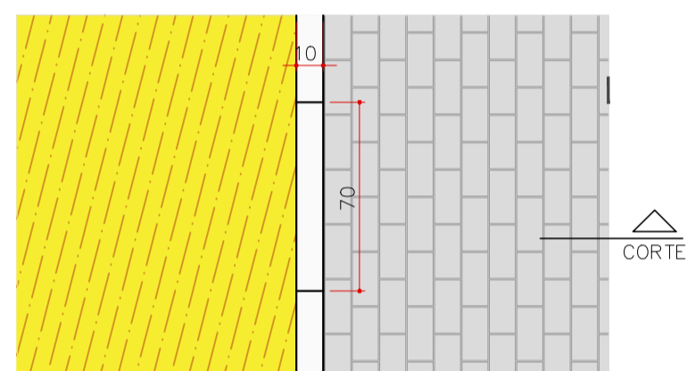
ENCONTRO DE PISOS - AREIA X INTERTRAVADO - E12 PLANTA ESCALA 1:25
