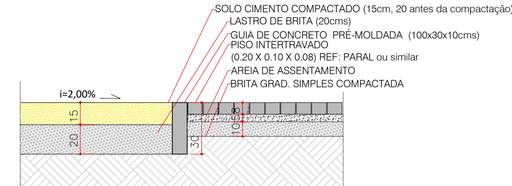
ENCONTRO DE PISOS - SOLO CIMENTO X INTERTRAVADO - E10 CORTE ESCALA 1:25
