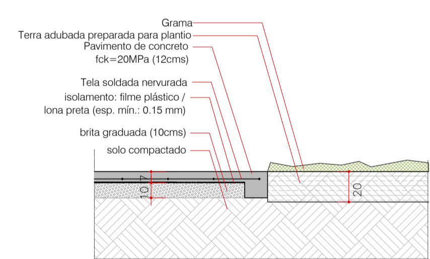
ENCONTRO DE PISOS - CONCRETO X GRAMA - E13 CORTE ESCALA 1:25
