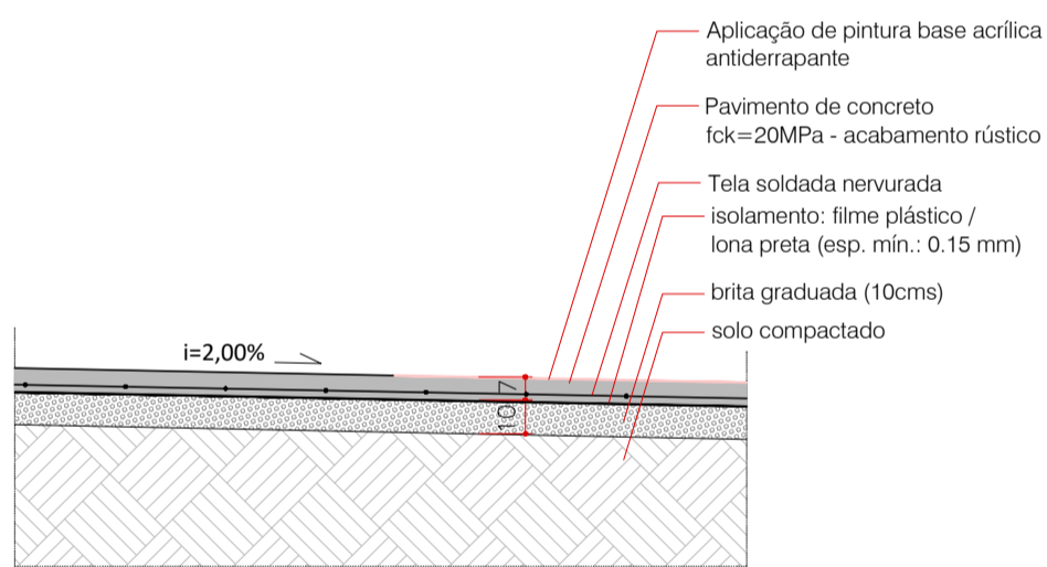
ENCONTRO DE PISOS - CONCRETO X CICLOVIA - E11 CORTE ESCALA 1:25
