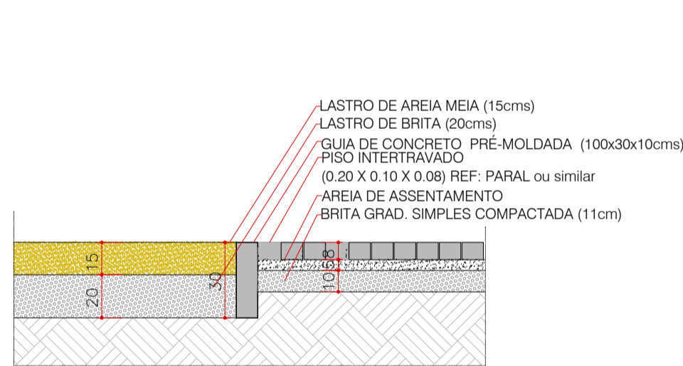
ENCONTRO DE PISOS - AREIA X INTERTRAVADO - E12 CORTE ESCALA 1:25
