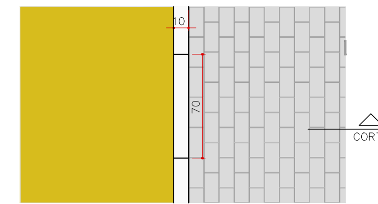
ENCONTRO DE PISOS - SOLO CIMENTO X INTERTRAVADO - E10 PLANTA ESCALA 1:25
