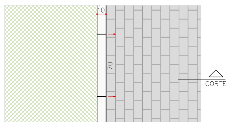
ENCONTRO DE PISOS - GRAMA X INTERTRAVADO - E15 PLANTA ESCALA 1:25
