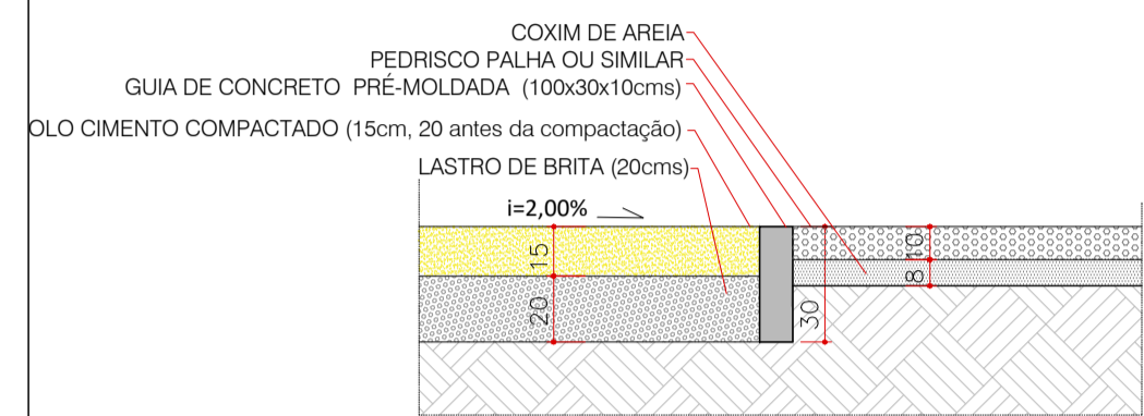
ENCONTRO DE PISOS - SOLO CIMENTO X GUIA X PEDRISCO - E7 CORTE ESCALA 1:25
