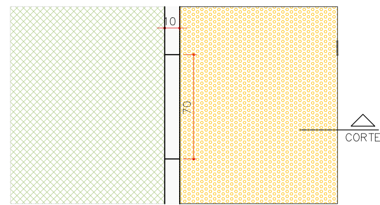
ENCONTRO DE PISOS - GRAMA X GUIA X PEDRISCO - E8 PLANTA ESCALA 1:25
