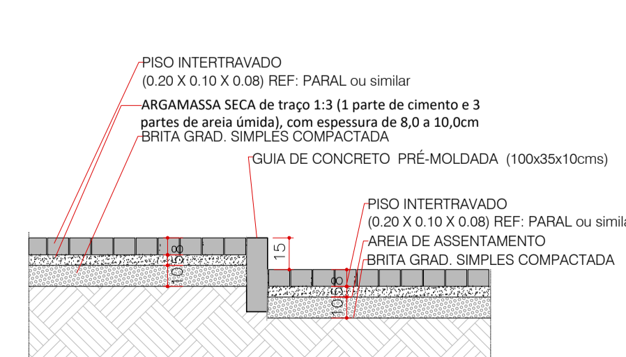
ENCONTRO DE PISOS - VIA DE INTERTRAVADO - E17 CORTE ESCALA 1:25
