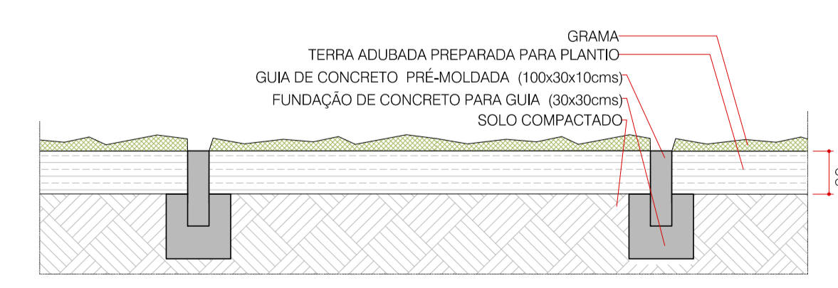
DETALHE DE GUIAS DE CONCRETO - DE1 CORTE B ESCALA 1:25
