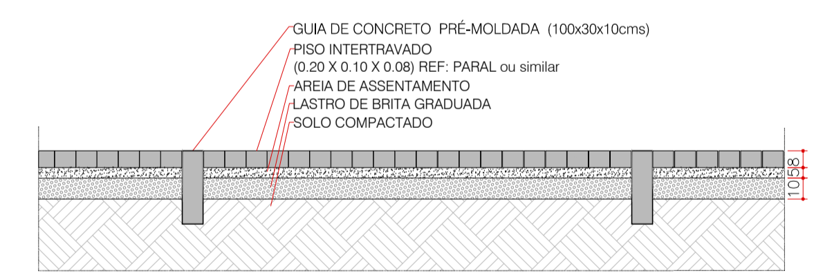
DETALHE DE GUIAS DE CONCRETO - DE1 CORTE A ESCALA 1:25
