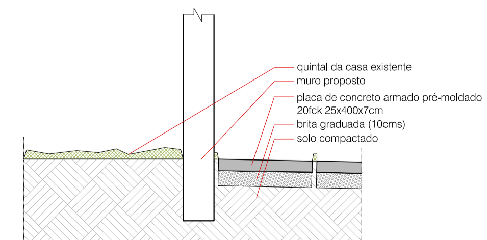
DETALHE DE ACESSO ÀS CASAS - E1 PLACA DE CONCRETO CORTE ESCALA 1:25
