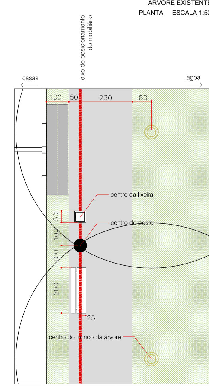
DETALHE DE POSICIONAMENTO - E1 BANCOS E LIXEIRAS NO PASSEIO DE FUNDO DE LOTE PLANTA ESCALA 1:100
