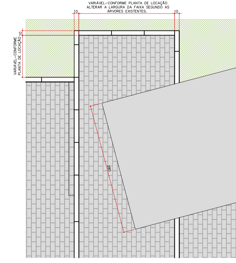
ENCONTRO DE PISO - DE1 CAMINHOS DE CONCRETO / PRAÇAS EM INTERTRAVADO PLANTA ESCALA 1:25
