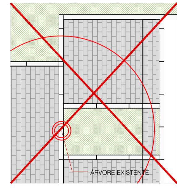
DETALHE DE DESENHO DE PISO - DE1 SITUAÇÃO NÃO DESEJÁVEL PLANTA ESCALA 1:50
