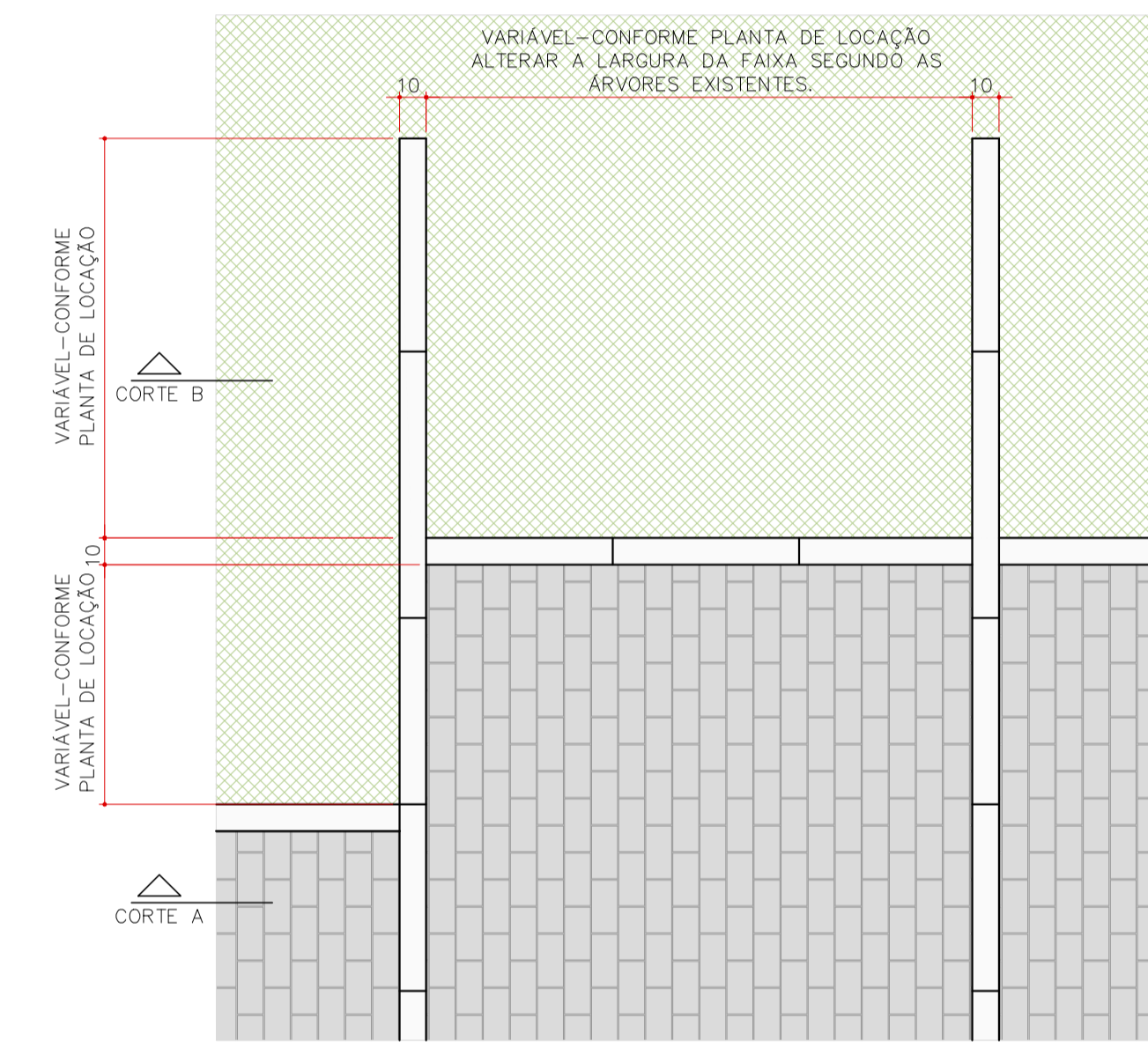
DETALHE DE GUIAS DE CONCRETO - DE1 PLANTA ESCALA 1:25
