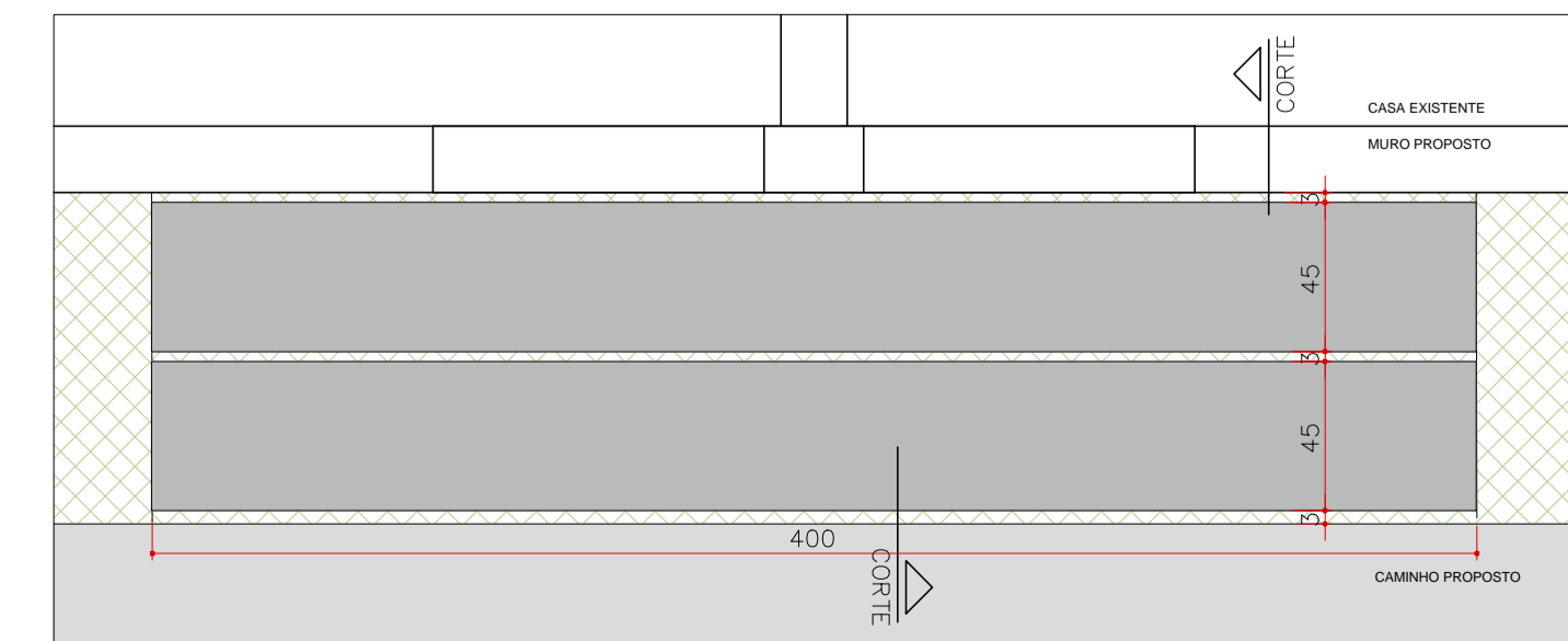
DETALHE DE ACESSO ÀS CASAS - E1 PLACA DE CONCRETO PLANTA ESCALA 1:25
