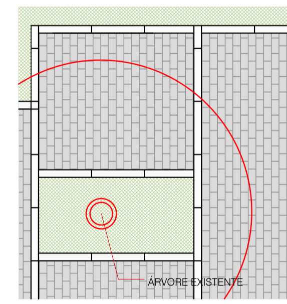
DETALHE DE DESENHO DE PISO - DE1 REDESENHO DO PISO - ADAPTAÇÃO À ÁRVORE EXISTENTE PLANTA ESCALA 1:50
