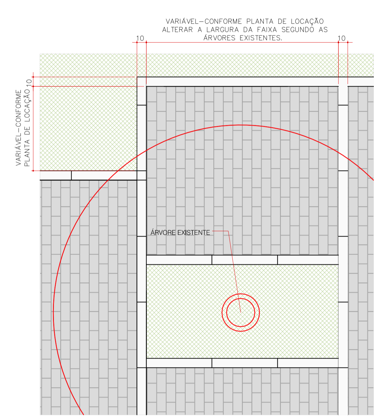
DETALHE DE DESENHO DE PISO - DE1 PLANTA ESCALA 1:25
