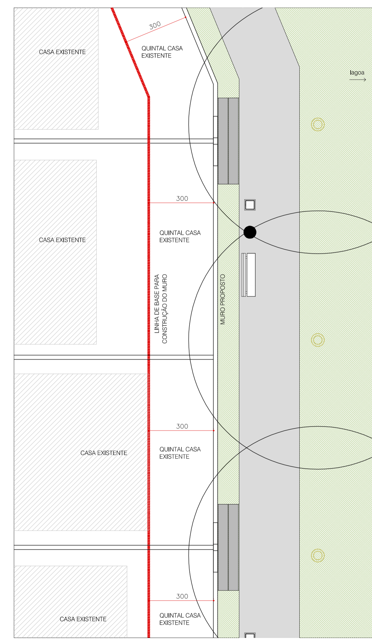
DETALHE DE CONSTRUÇÃO DO MURO - E1 EM RELAÇÃO ÀS CASAS EXISTENTES
