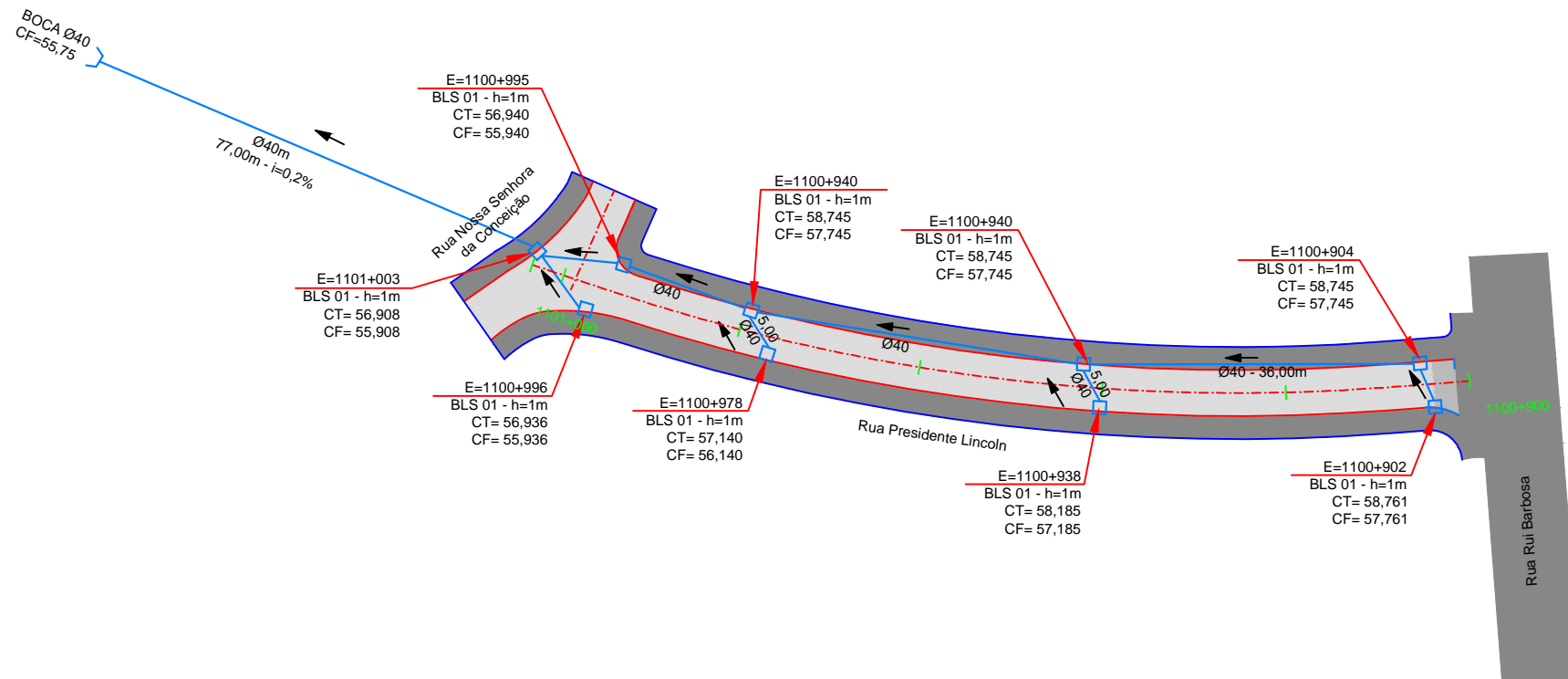
PLANTA DE DRENAGEM - ESQUEMÁTICA ESCALA 1:750
